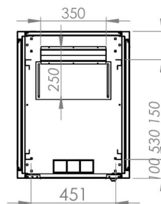
Vue détaillée
