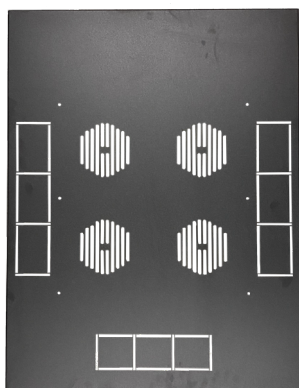
Toit : passage de câbles sur les 4 côtés
